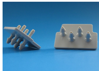
Spritzgewicht: 6,5 g Kunststoff: POM Minibohrungen durch die Kanülen
