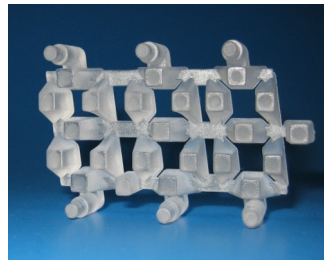
Spritzgewicht: 10,8 g Kunststoff: PC Spezielle optische Fläche
