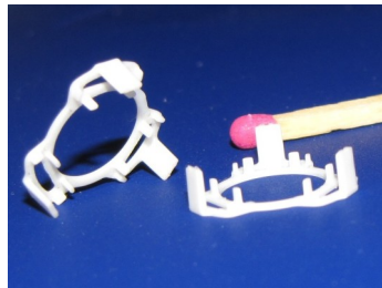
Spritzgewicht: 1 g Kunststoff: PBT 50% GF Unser kleinster Teil
